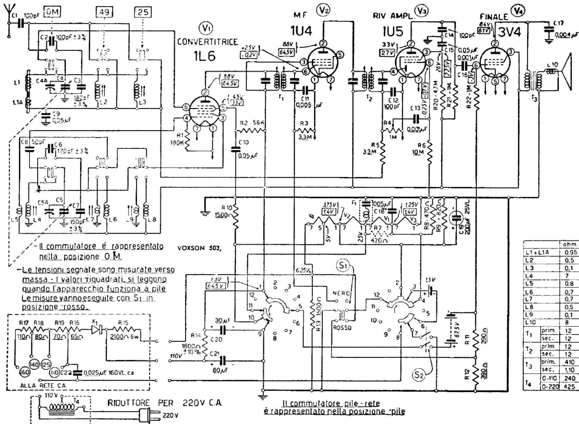
FARET - Portatile Voxson mod. 503 Dinghy I serie. Funziona con pile interne o con alimentatore separato a selenio in corrente alternata. Gamme d'onda: medie da 520 a 1600 kc. Corte da 5,9 a 6,3 Mc. Cortissime da 11,4 a 12,3 Mc. Commutatore di gamma a pulsanti. Telaio interno, antenna a stilo per OC. Media frequenza 455 kc. Uscita 25-30 mW.
